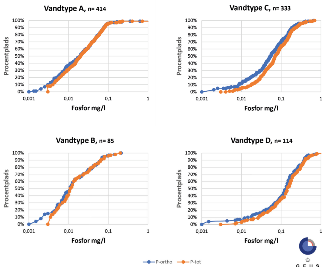
Figur 43. GRUMO. Koncentrationsfordelingen for det gennemsnitlige fosforindhold i GRUMO-indtag for re- doxvandtype A-D for P_{tot} og P_{ortho} for perioden 2019-2020. Antal indtag (n) for hver re- doxvandtype. Bemærk, der er anvendt en logaritmisk skala.
