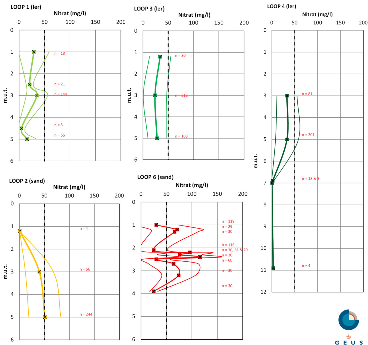
Figur 28. LOOP. Gennemsnitlig nitratkoncentration i grundvand i LOOP-indtag opgjort på filterdybder (indtagetets top) i m u.t. for lerjords- og sandjordsoplandene i perioden 2016-2020. Gennemsnittet er baseret på alle målinger i det angivne dybdeniveau. Spredningen (standardafvigelsen) omkring gennemsnittet er angivet med tyndere streg. Antallet af målinger (n) er vist for hver dybde.
