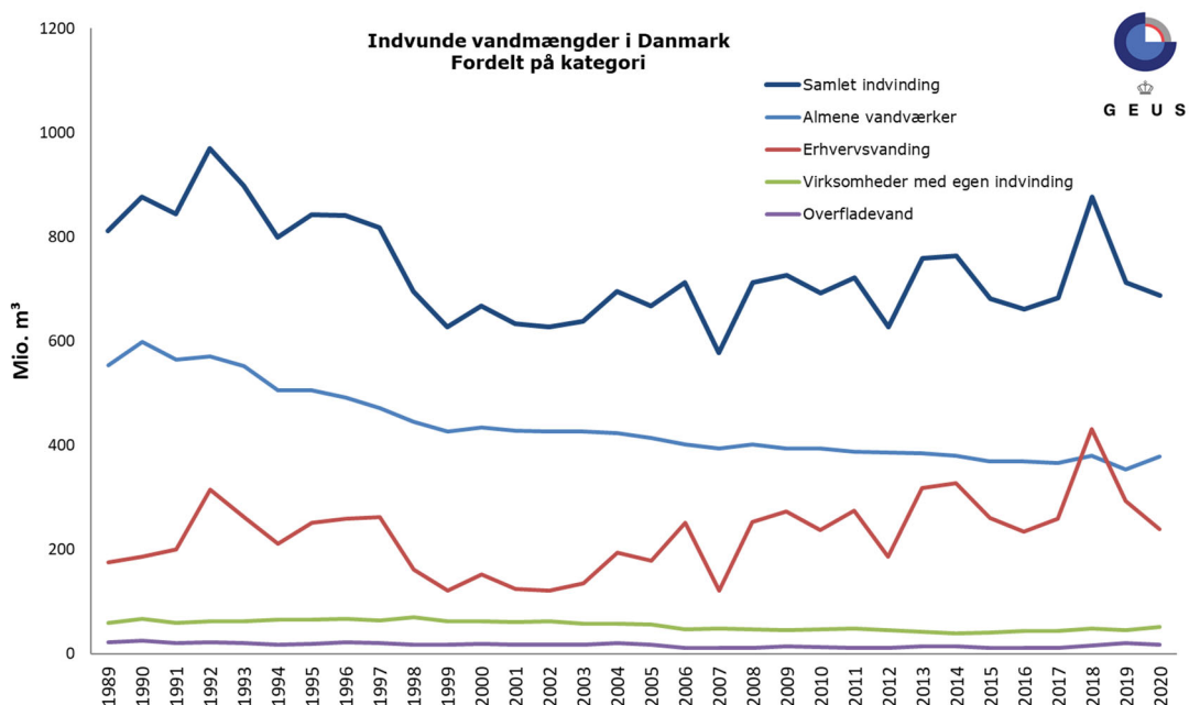
Figur 1. Vandindvinding i Danmark i perioden 1989-2020 opdelt på almene vandværker, erhvervsvand, industri og overfladevand. Med en fed, mørkeblå linje er den samlede indberettede indvinding vist. Bemærk, hvorledes den varierer med erhvervsvandingen, hvoraf markvandingen udgør hovedparten.
