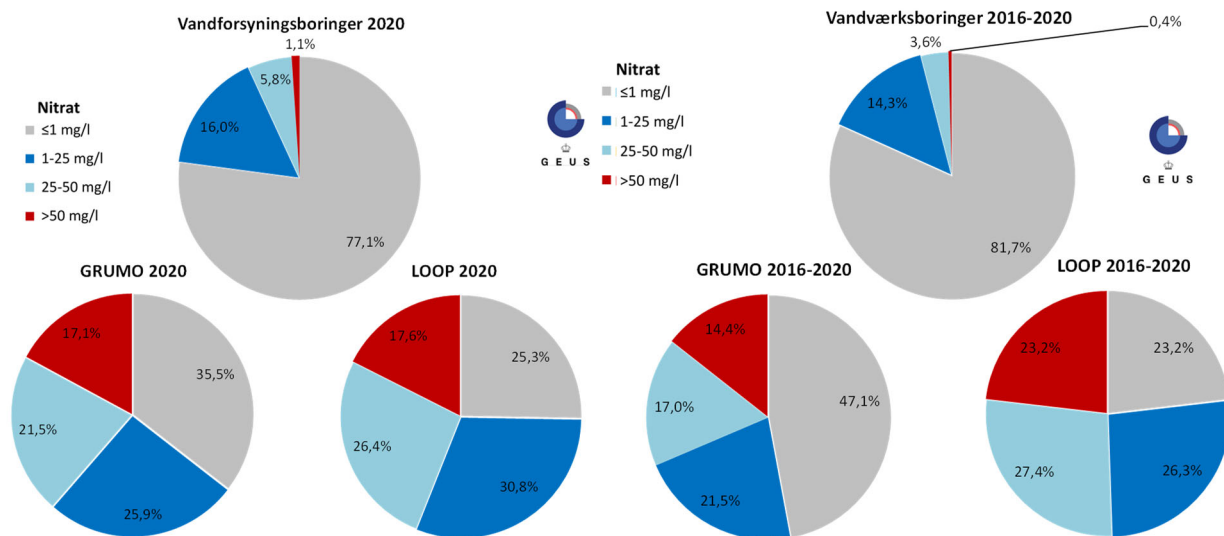
Figur 22. GRUMO, LOOP & Vandforsyning. Fordelingen af det gennemsnitlige nitratindhold pr. indtag i 2020 for 806 GRUMO-indtag, 91 LOOP-indtag og 1.607 vandforsyningsboringer og i perioden 2016-2020 for 1.277 GRUMO-indtag, 95 LOOP-indtag og 6.111 vandforsyningsboringer.
