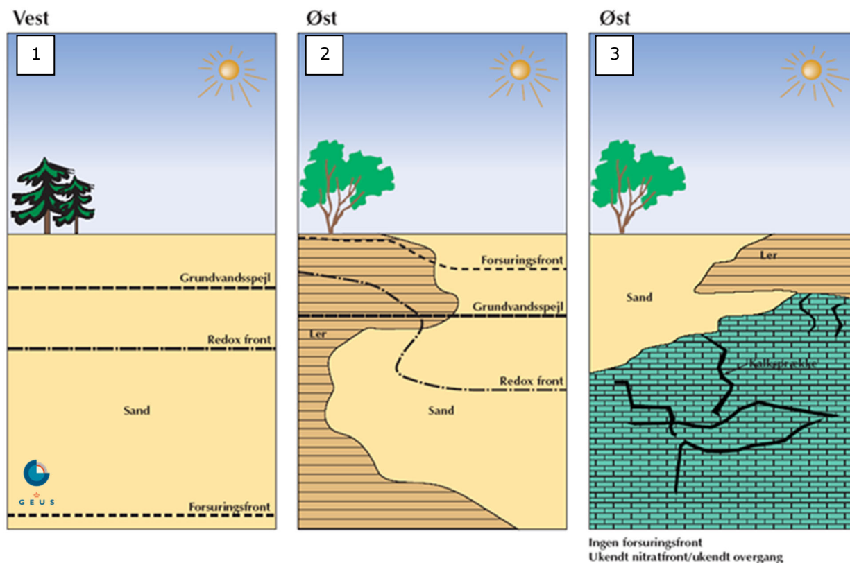
Figur 79. Principskitse over beliggenheden af forsøringsfronten og redoxfronten i tre typiske geologiske situationer: 1) Vestdanmark, hvor jordlagene overvejende består af sand, 2) Østjylland, Fyn og Vestsjælland, hvor geologisk heterogenitet med vekslende ler og sand giver store lokale variationer i dybden til fronterne og 3) områder med kalklag, fx Stevns og omkring Ålborg (Figur 73), hvor sprækkedannelser gør fastlæggelse af nitratfronten i selve kalklagene svær at forudsige. Bemærk, at forsøringsfronten kan ligge både over og under redoxfronten.
